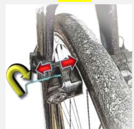
Abstand von 1–2 mm einstellen (mit kleinem Inbusschlüssel)
